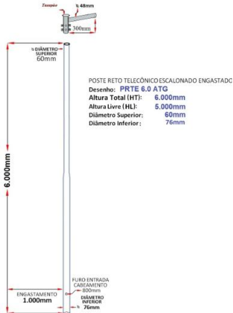
Figura 2 – Poste para Iluminação Pública.
