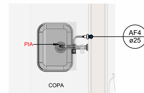
DT02- COPA SUBSOLO Escala: 1 : 20
