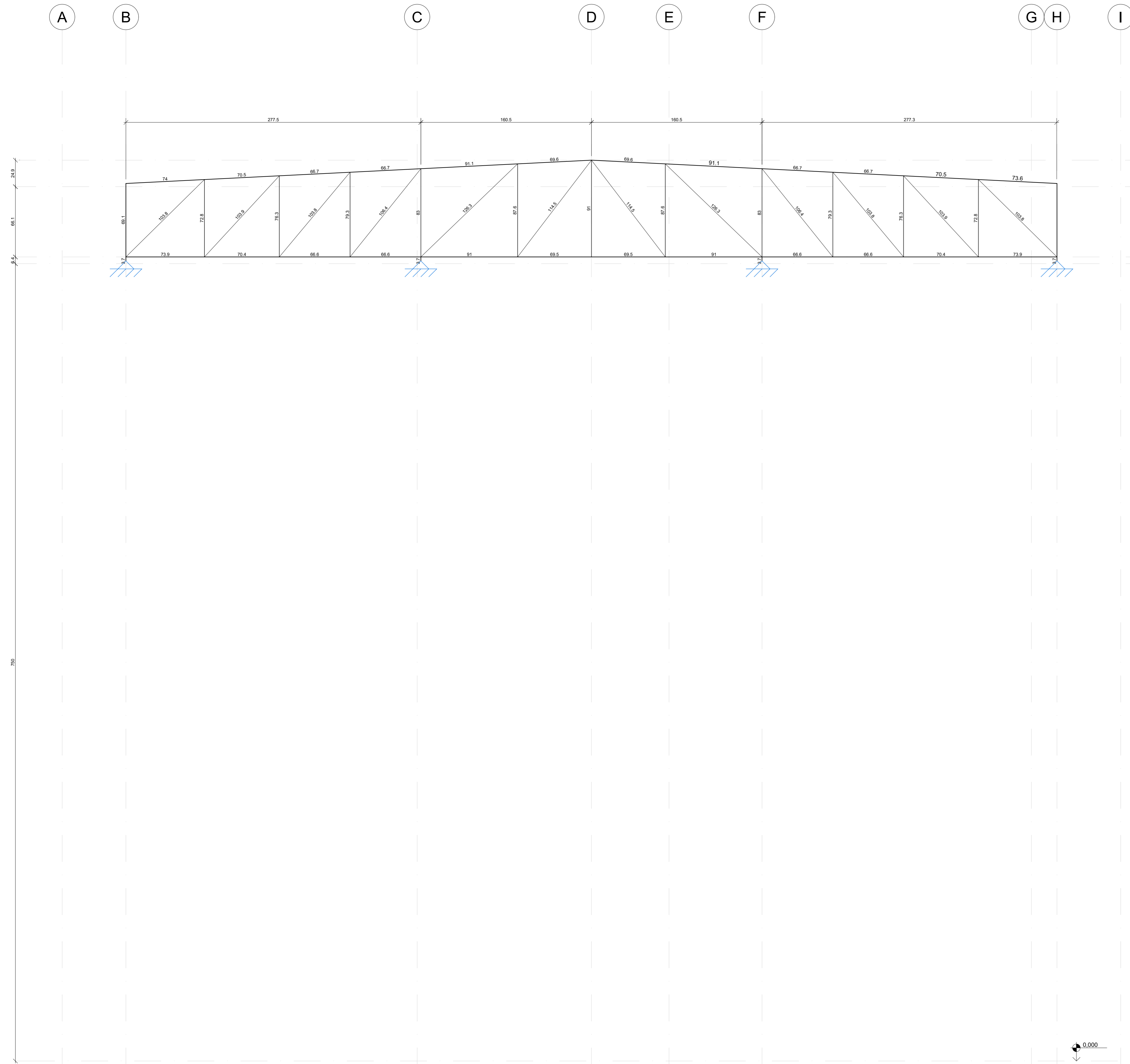
VISTA - DIMENSÕES - EIXO 3 @ 5 Esc. 1:20
