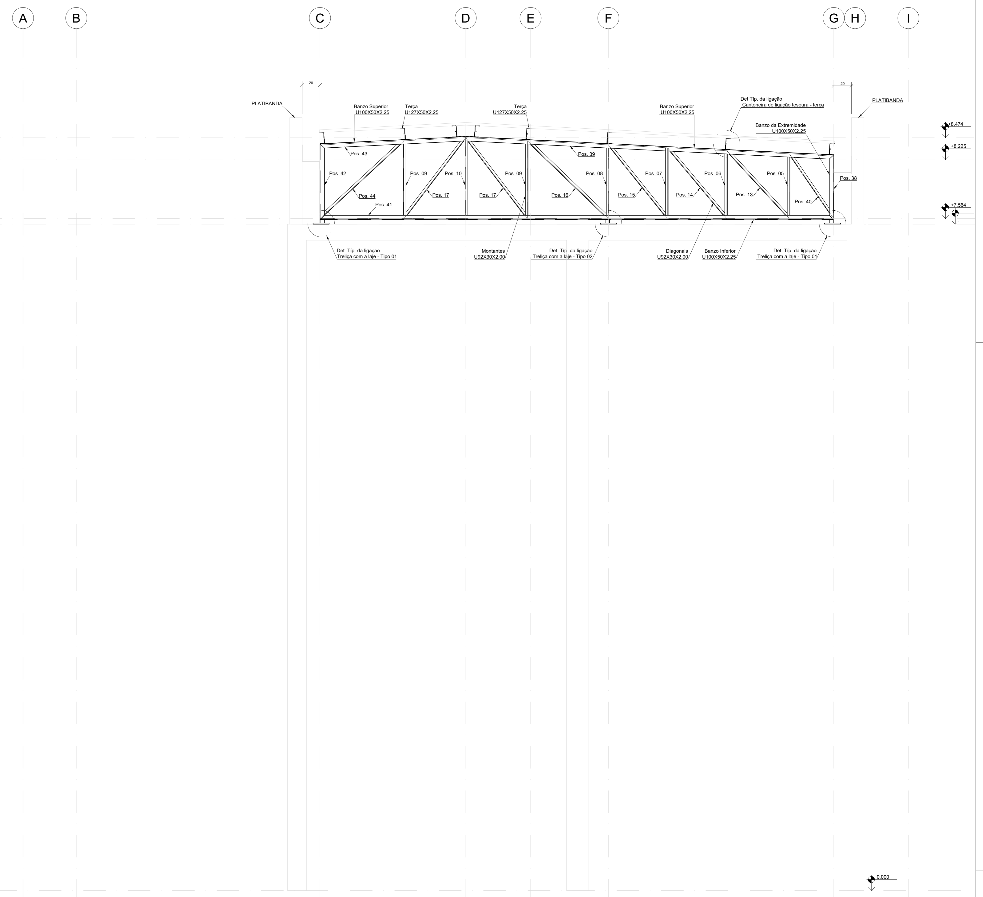
VISTA - EIXO 9 Esc. 1:20
